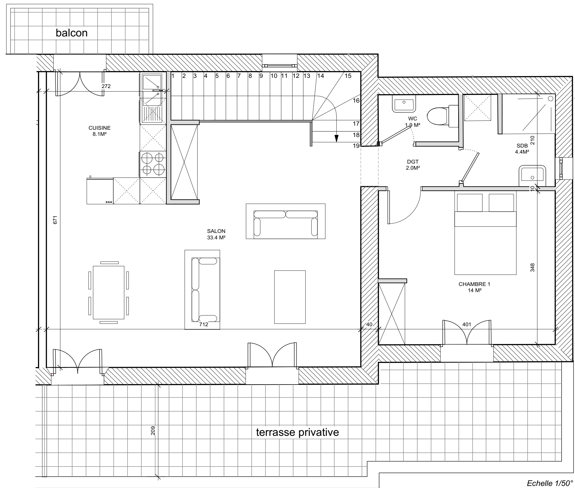
PLAN DE L'ENTREE AU RDC
