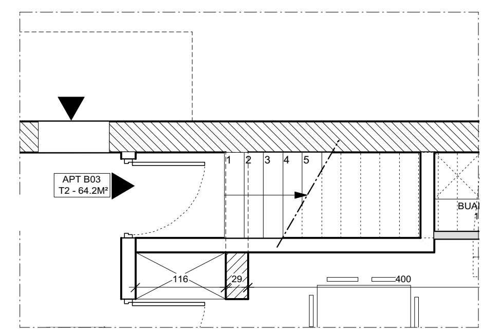
PLAN DE L'ENTREE AU RDC
