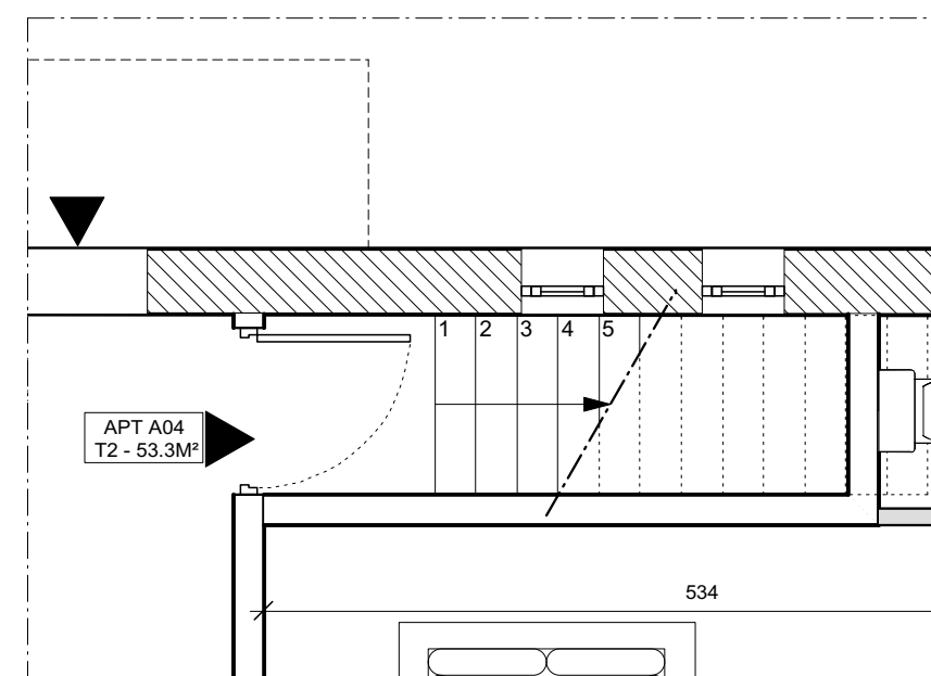
PLAN DE L'ENTREE AU RDC
