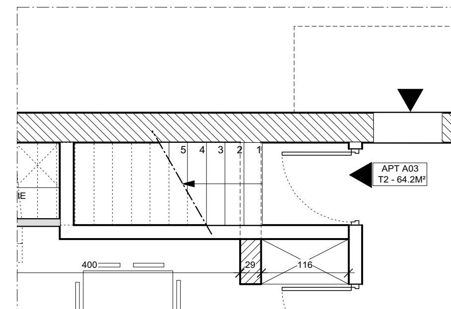
PLAN DE L'ENTREE AU RDC
